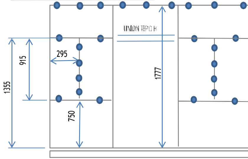
ESQUEMA ORIENTATIVO PARA ELIACION DE TORNILLOS PARA AFIRMAR EL FONDO DE PLACARD
